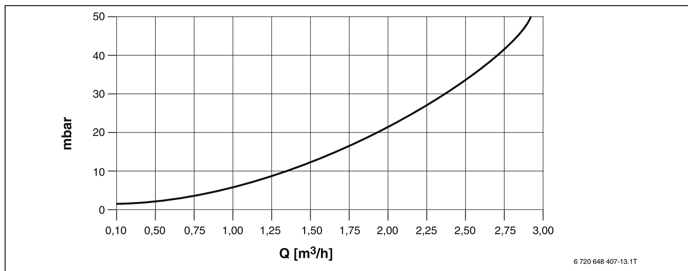
Рис. 5 Гидравлические потери давления (мбар) в зависимости от объёмного расхода ( m^3/h )
