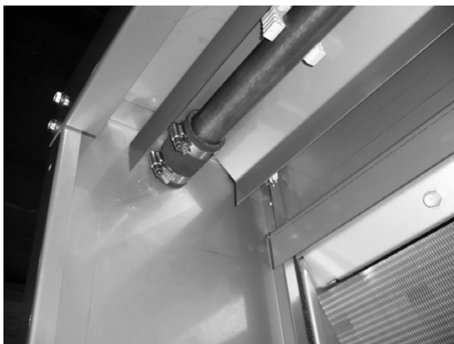
Рисунок 16: Соединение гибкого рукава с зажимами
