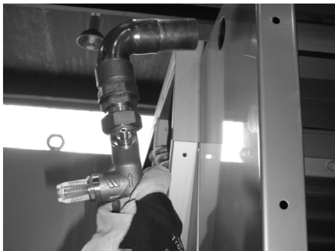
Рисунок 7: Подсоединение подачи воды
