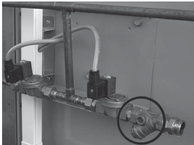
Рисунок 4: Водяной фильтр
