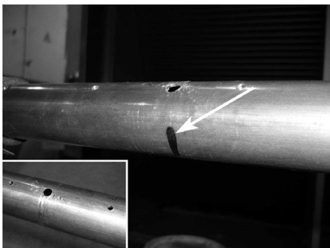
Рисунок 11: Совместительное отверстие
