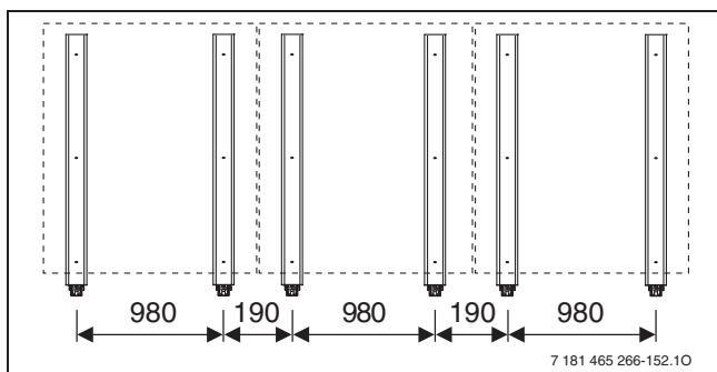
Рис. 156 Исполнение для максимальной нагрузки, 3 вертикальных коллектора
