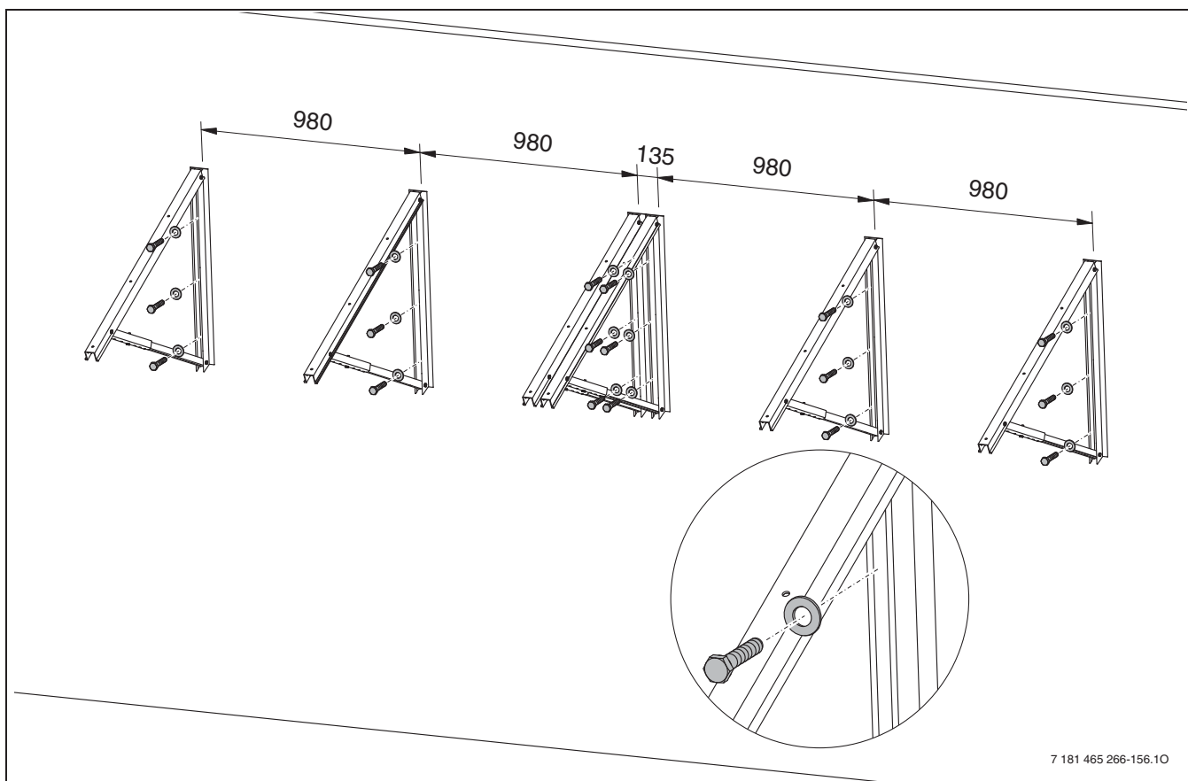
Рис. 164 Расположение опор на фасаде для двух коллекторов
