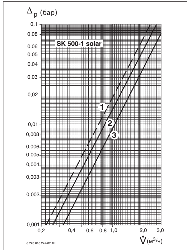
Рис. 56 Потери давления WST SK 500-1 solar
