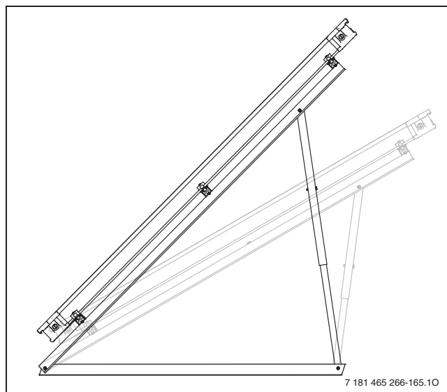
Рис. 151 Установочный угол коллектора на плоской крыше
