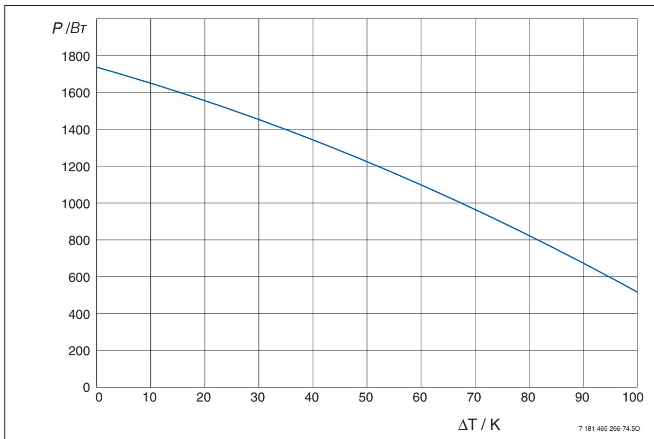
Рис. 45 Мощность плоского коллектора FKS-1 при интенсивности излучения 1000 \text{ Вт/м}^2
