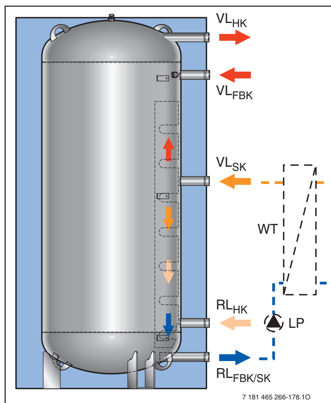
Рис. 29 Бак-накопитель
