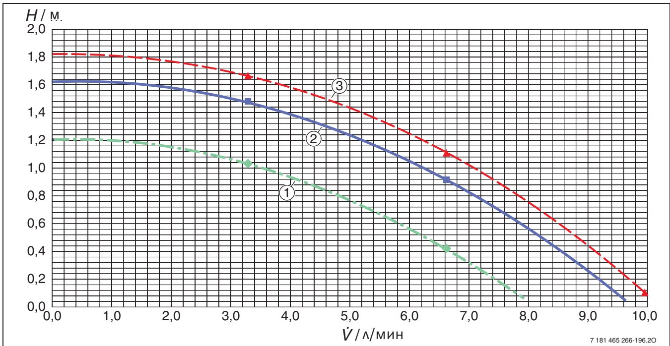
Рис. 110 Остаточная высота подачи циркуляционного насоса
