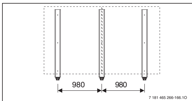
Рис. 161 Основное исполнение для 2 вертикальных коллекторов
