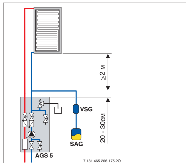
Рис. 94 Установка предвключённый охладительный резервуар
