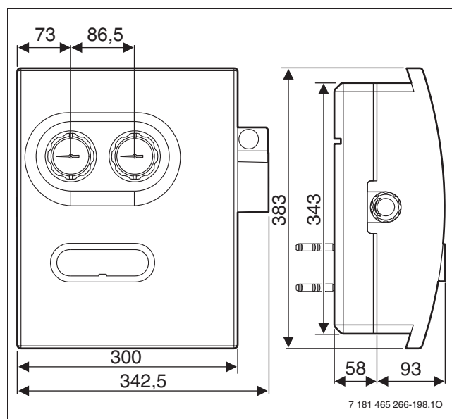
Рис. 109 Размеры
