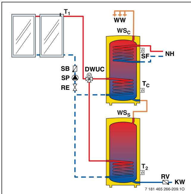
Рис. 73 Схема с приоритетным бойлером С и следующим геолобойлером
