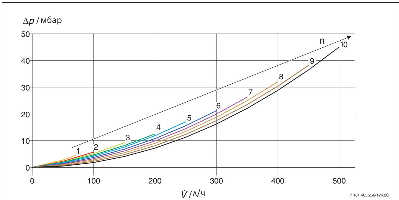
Рис. 44 Потери давления плоского коллектора FKC-1S (объёмное соотношение воды и гликоля 55/45 %)
