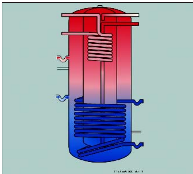
Рис. 28 Комбинированный гелиобойлер
