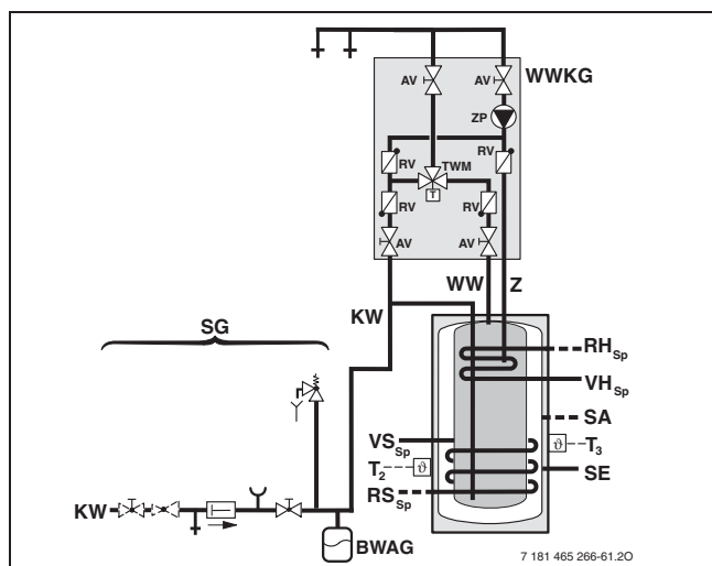
Рис. 48 Схема подключения контура ГВС с поддержкой отопления от солнечного коллектора с группой комфортного режима ГВС
