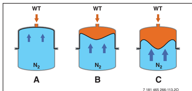
Рис. 35 Принцип действия мембранного расширительного бака (MAG)
