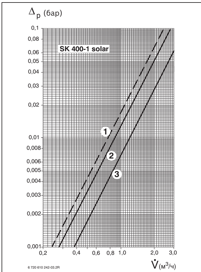
Рис. 55 Потери давления WST SK 400-1 solar
