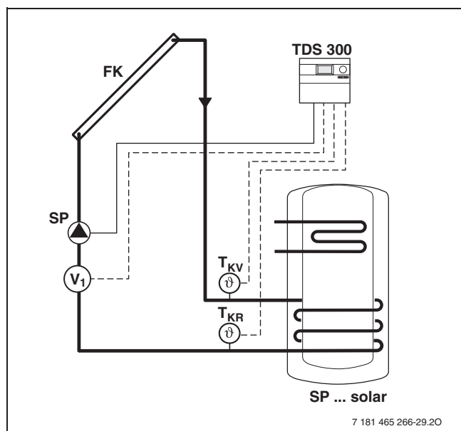
Рис. 78 Схема подключения теплового счётчика
