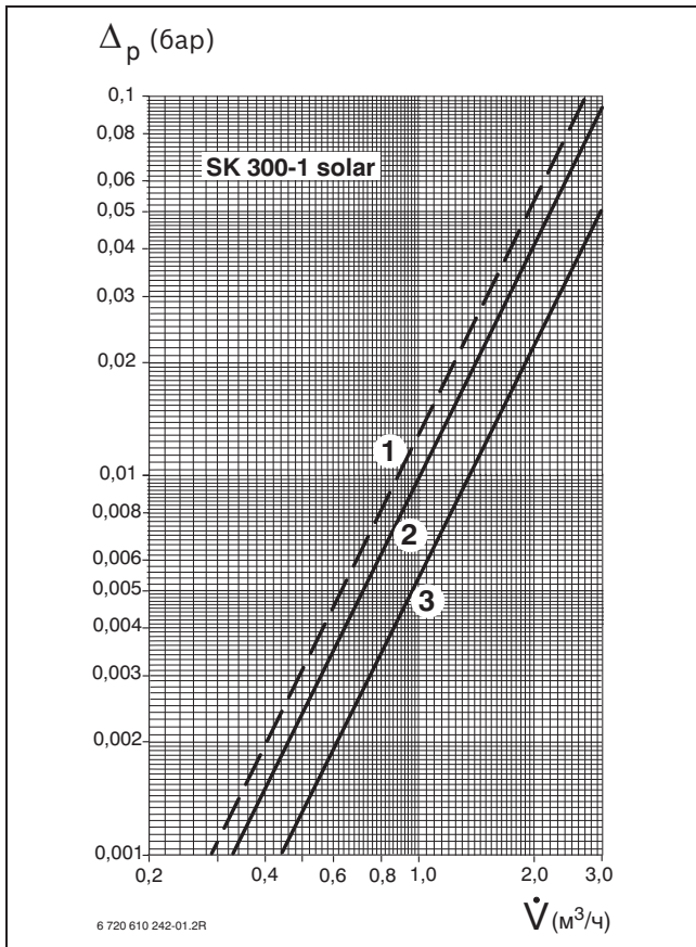
Рис. 54 Потери давления WST SK 300-1 solar
