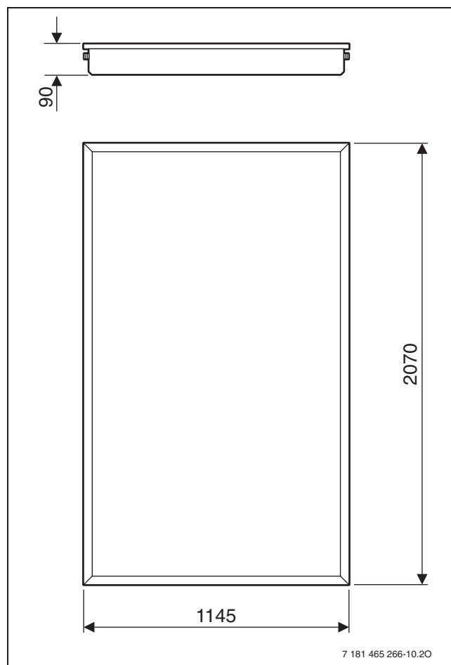
Рис. 42 Габаритные размеры FKC-1
