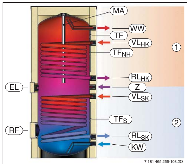
Рис. 27 Гелиобойлер
