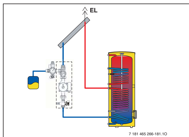
Рис 36 Схема с одноконтурной насосной станцией и воздухоотделителем на крыше
