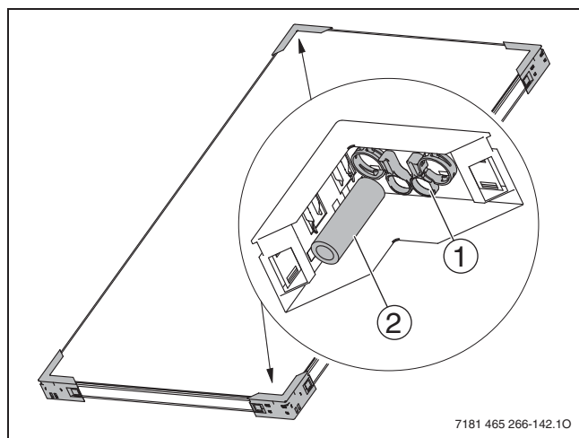
Рис. 141 Два транспортировочных уголка с соединительными комплектами (здесь FKC-1)
