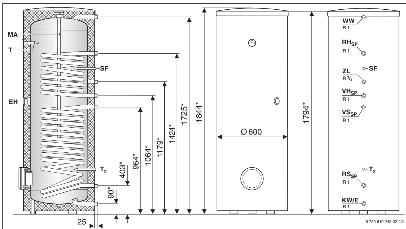
Рис. 52 Габаритные и присоединительные размеры WST SK 300-1 solar
