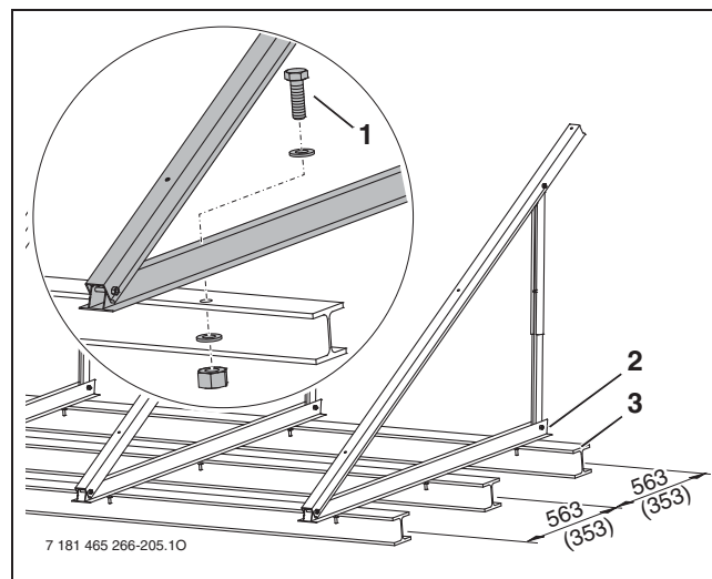
Рис. 158 Подставки для плоской крыши, закреплённые на двутавровых балках, размеры в мм (значения в скобках = для горизонтального исполнения)
