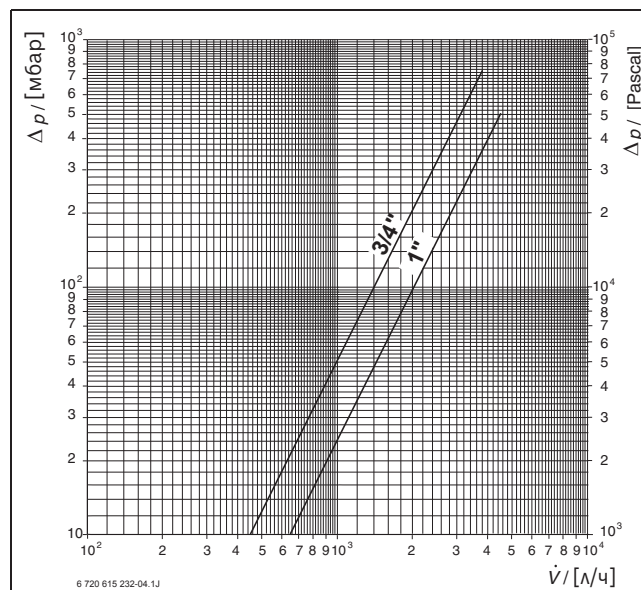
Рис. 105 Потери давления DWU 20 и DWU 25 (вода)
