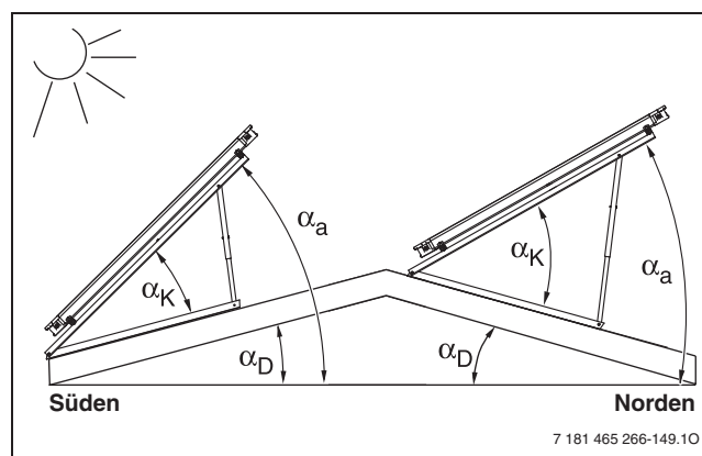
Рис. 153 Угол установки на наклонных крышах
