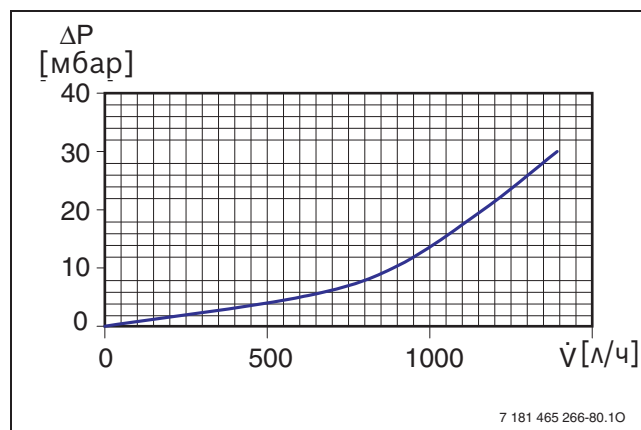
Рис. 98 Потери давления ELT (вода)
