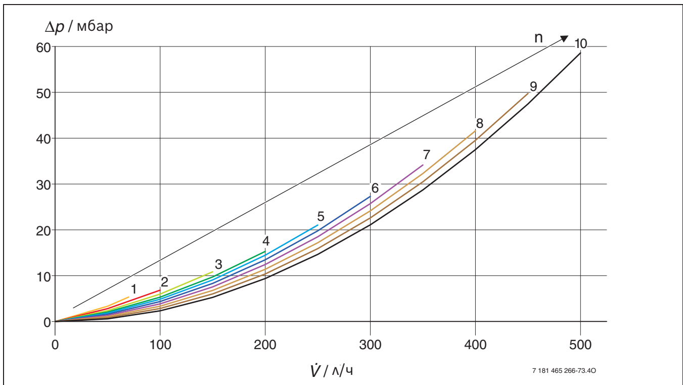
Рис. 43 Потери давления плоского коллектора FKC-1W (объёмное соотношение воды и гликоля 55/45 %)
