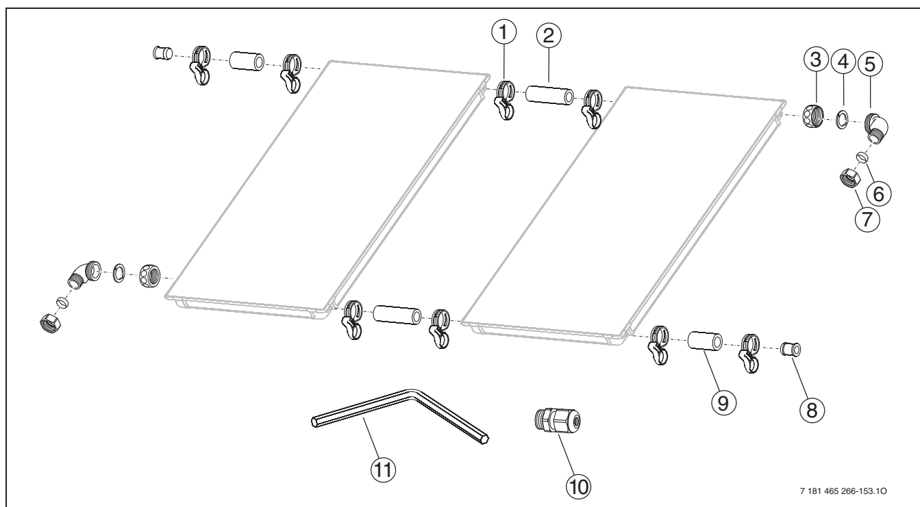
Рис. 149 Комплект подключения и соединительный комплект для FKC-1
