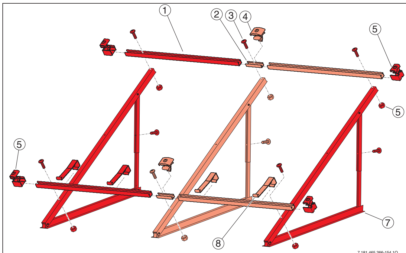
Рис. 150 Основной и дополнительный монтажные комплекты для установки на плоской крыше
