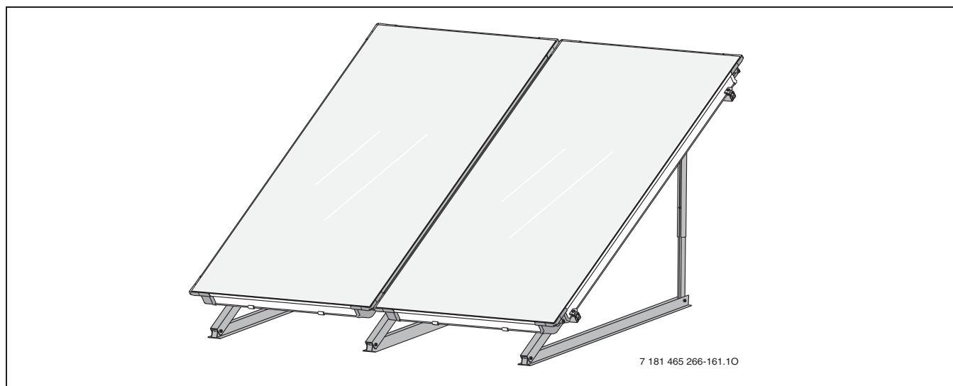
Рис. 148 Монтаж на плоской крыше двух плоских коллекторов FKC-1S
