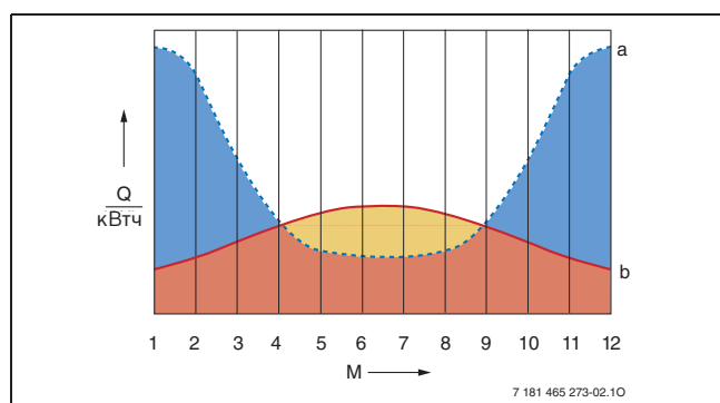
Рис. 5 Энергия, вырабатываемая солнечной установкой, и потребности в энергии для отопления и горячего водоснабжения
