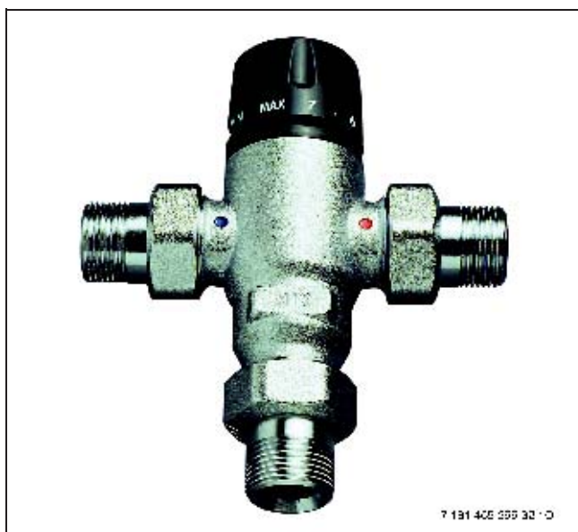
Рис. 106 TWM
