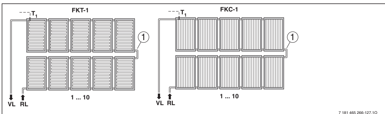
Рис. 128 Последовательное соединение солнечных коллекторов в два ряда
