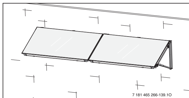
Рис. 140 Монтаж на фасаде
