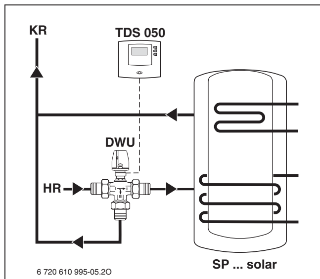
Рис. 104 Поддержка отопления нагревом от контура солнечного коллектора с бойлером SP... solar
