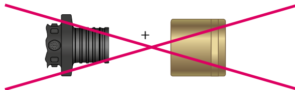
Рис. 16 Недопустимая комбинация фитинга RAUTITAN PX с подвижной гильзой RAUTITAN MX
