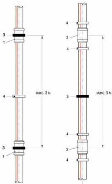
Рис. 76 Применение двухраструбных или подвижных муфт
