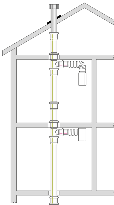
Рис. 56 Система вытяжной вентиляции из труб RAUPIANO PLUS
