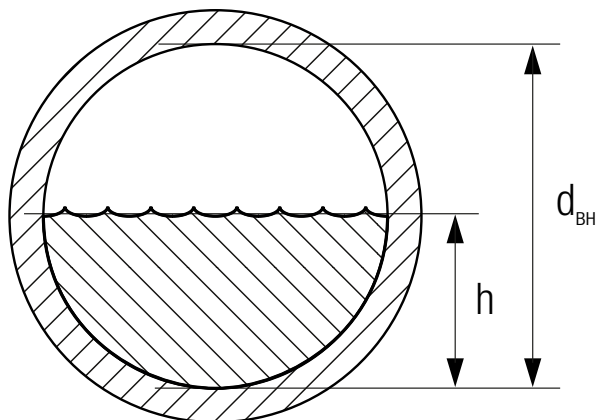
Рис. 91 Поперечный разрез частично наполненного трубопровода d_{вн} Внутренний диаметр трубы h Высота жидкости
