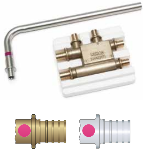
Рис. 20 Отличительные особенности фитингов для систем отопления
