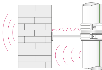
Рис. 67 Снижение шума в системе RAUPIANO PLUS
