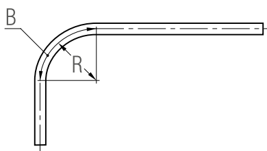
Рис. 46 Обозначение радиуса и длины изгиба R = радиус изгиба B = длина изгиба
