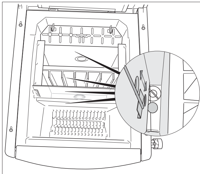
Рис. 34 Чистка стенок
