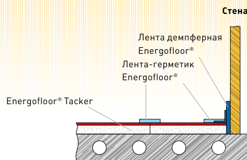
Бетонное основание
