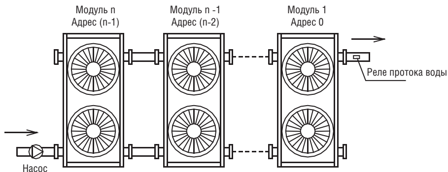
Рис. 4-9 (менее 6 модулей)
