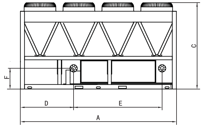
Вид спереди
