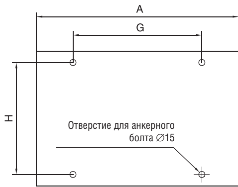
Вид снизу
