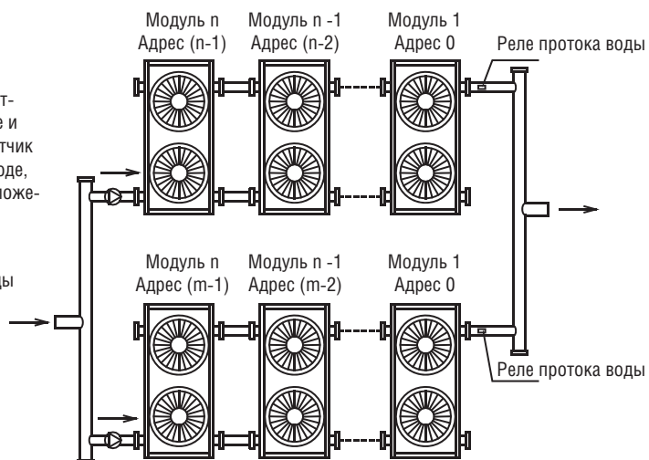
Рис. 4-12 (монтажная схема: менее 16 модулей)
