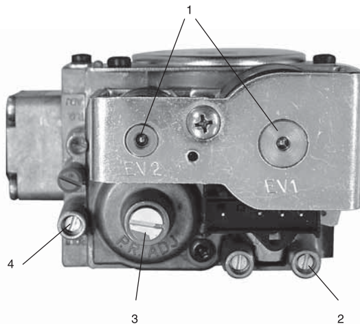
Рис. 17: Газовый клапан
