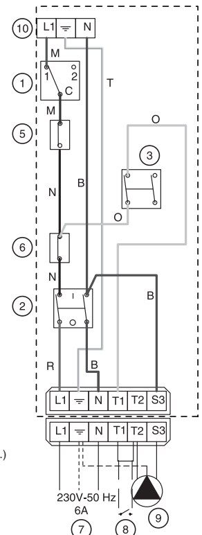
Рис. 9: Управляющая электрическая схема
