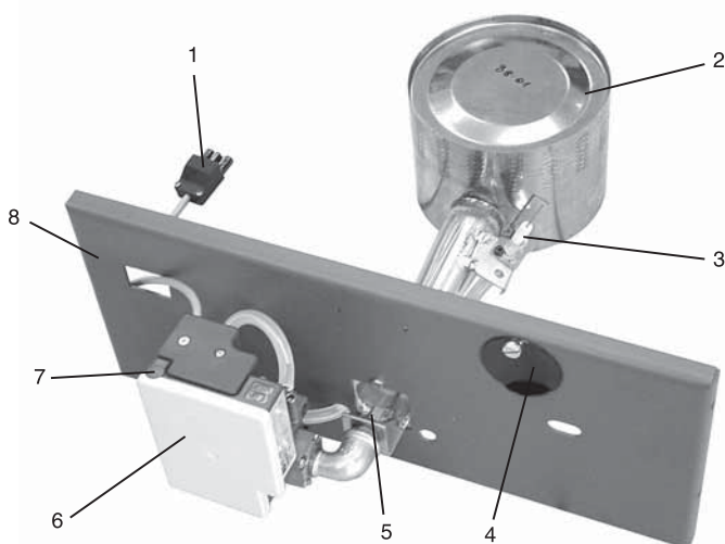
Рис. 18: Атмосферная газовая горелка на пропане
