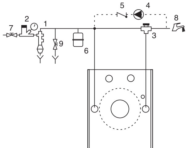
Рис. 5б: Схема с термостатическим смесителем.
