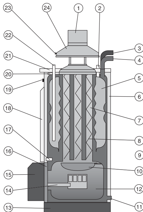
Рис. 15: Устройство котла
