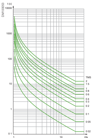
Кривая длительной обратно-зависимой выдержки времени МЭК (МЭК/LTI)
