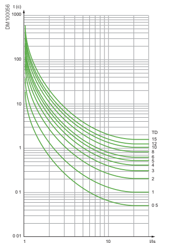
Кривая сильно обратно-зависимой выдержки времени IEC (IEE/EI или МЭК/F)
