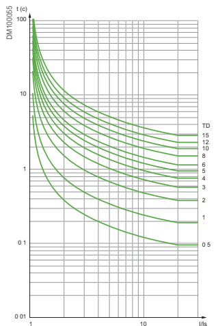
Кривая умеренно обратно-зависимой выдержки времени IEC (IEE/MI или МЭК/D)
