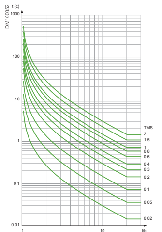
Кривая сильно обратно-зависимой выдержки времени МЭК (МЭК/VIT или МЭК/B)
