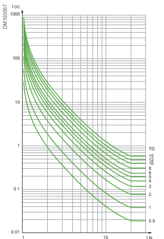
Кривая чрезвычайно обратно-зависимой выдержки времени IEC (IEE/VI или МЭК/E)
