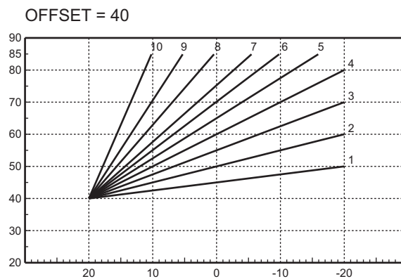
fig. 12 - Ejemplo de desplazamiento paralelo de las curvas de compensaci3n
