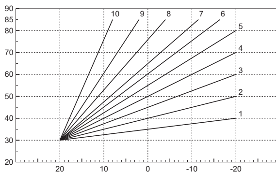
fig. 11 - Curvas de compensaci3n
