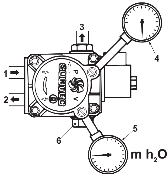
fig. 21 - Bomba
