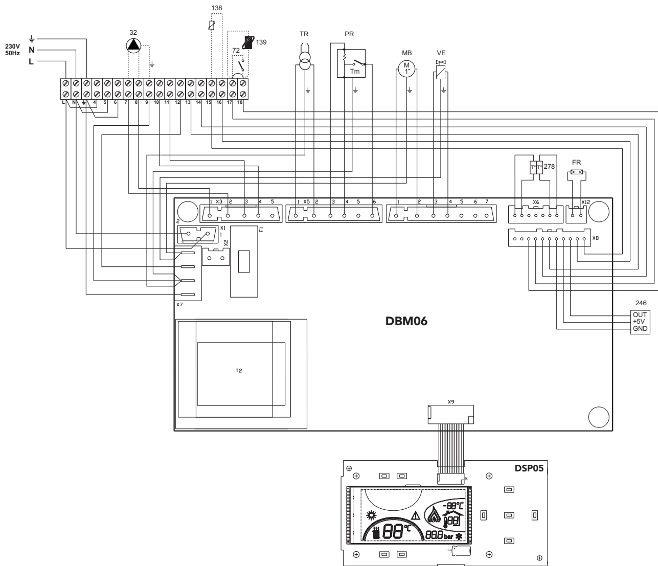
fig. 33 - Esquema eléctrico
