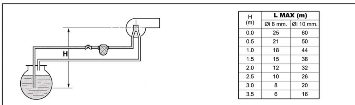
fig. 16 - Alimentación por aspiración
