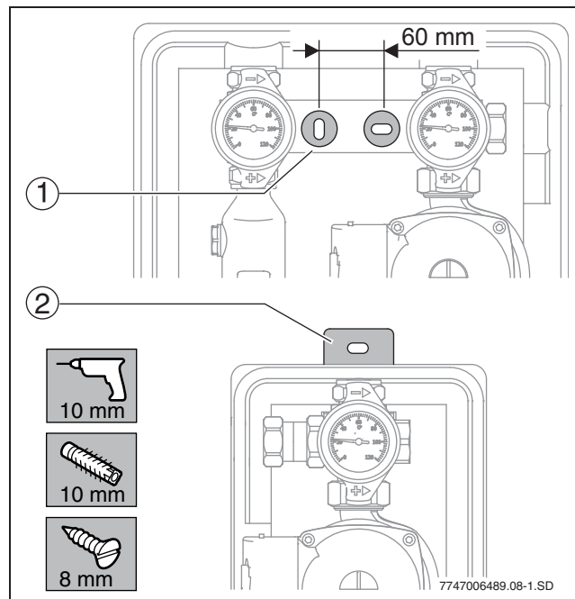
Рис. 7 Монтаж станции
