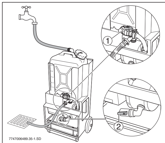
Рис. 22 Промывка насоса и бака
