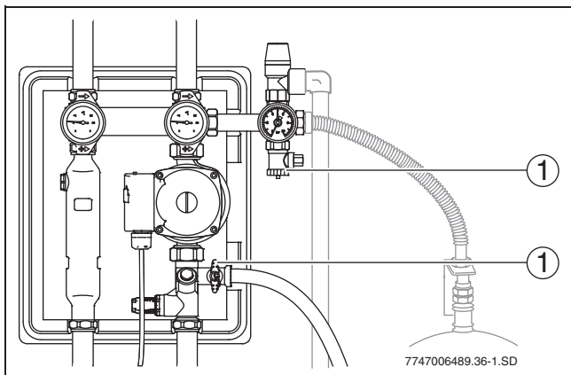
Рис. 27 Заполнение через кран для заполнения и слива
